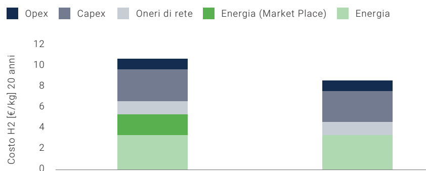
Figura 43 LCOH con orizzonte temporale di 20 anni e costo energia con (a sinistra) e senza (a destra) la quota relativa al valore di mercato
