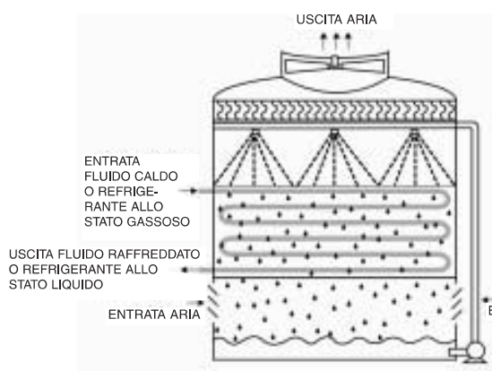
Figura 5 - Tiraggio Indotto
