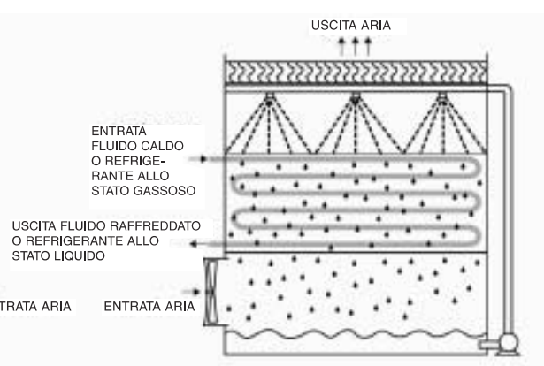
Figura 6 - Tiraggio forzato
